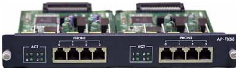
AP-FXS8 Module
